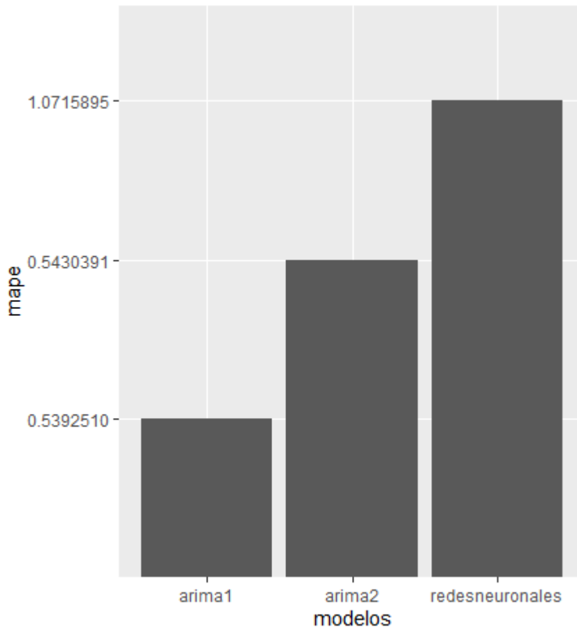
Gráfico 10: (DJI) comparativo modelos y MAPE.
