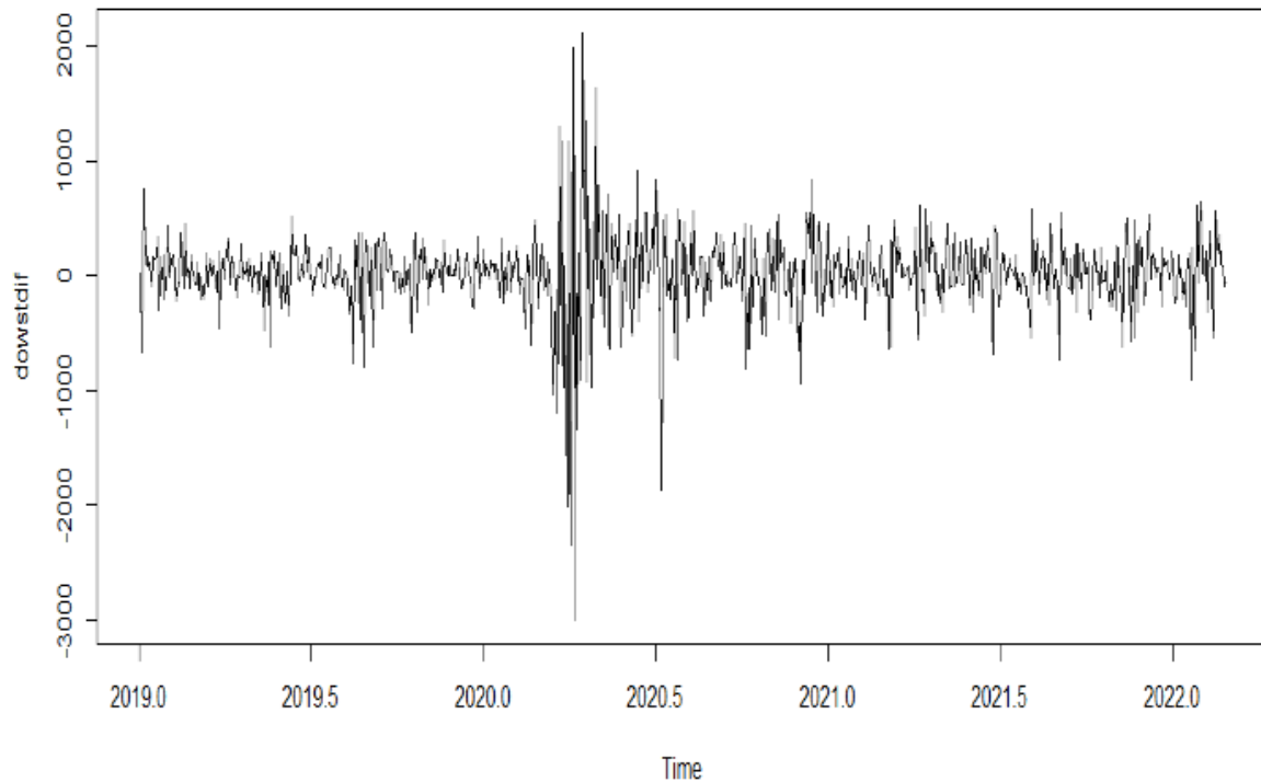
Gráfico 3: (DJI) Test Dickey Fuller
