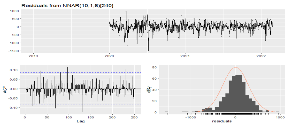
Gráfico 7: (DJI) residuales modelo red neuronal.
