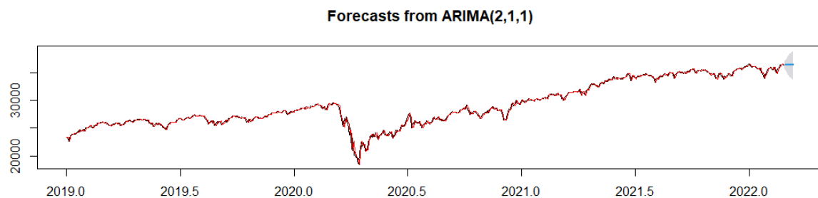
Gráfico 7: (DJI) pronostico modelo ARIMA modelo 2.
