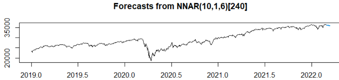
Gráfico 8: (DJI) pronostico del modelo neuronal.
