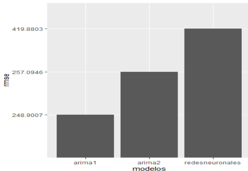
Gráfico 9: (DJI) comparativo modelos y RMSE.
