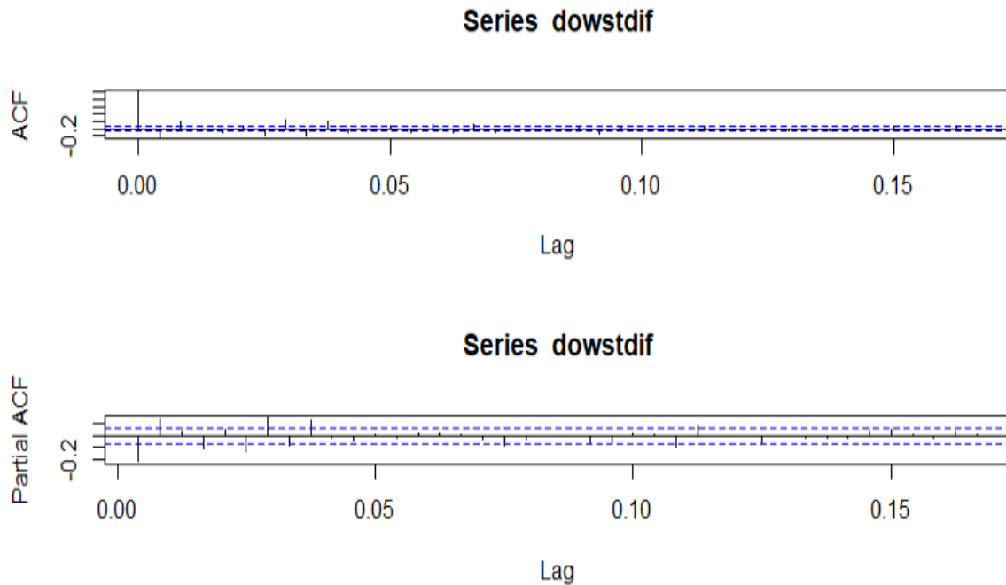
Gráfico 4: (DJI) autocorrelación y autocorrelación parcial.
