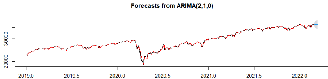
Gráfico 6: (DJI) pronostico modelo ARIMA modelo 1.
