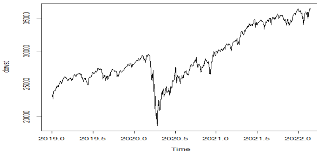
Grafico 1: (DJI) serie de tiempo entre los tiempos comprendidos de estudio.
