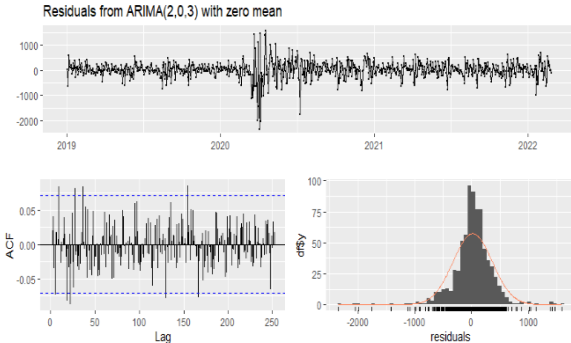
Gráfico 5: (DJI) Residuales Modelo ARIMA.
