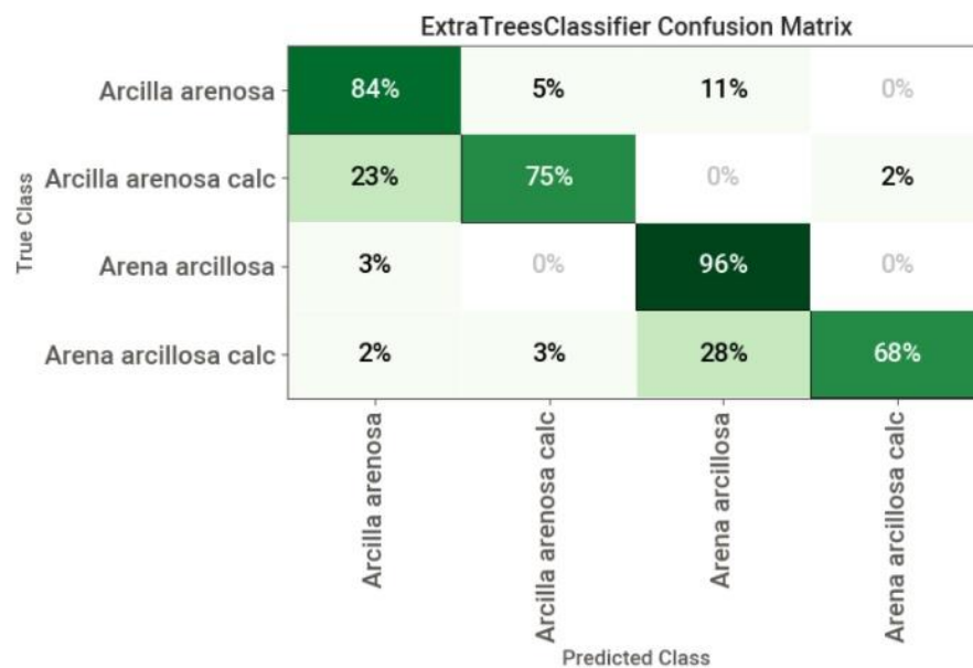
Figura 3. Matriz de Confusión para Problema 2 . Se observa una visible disminución en los porcentajes de predicción, sobre todo para la clase Arena arcillosa calcárea
