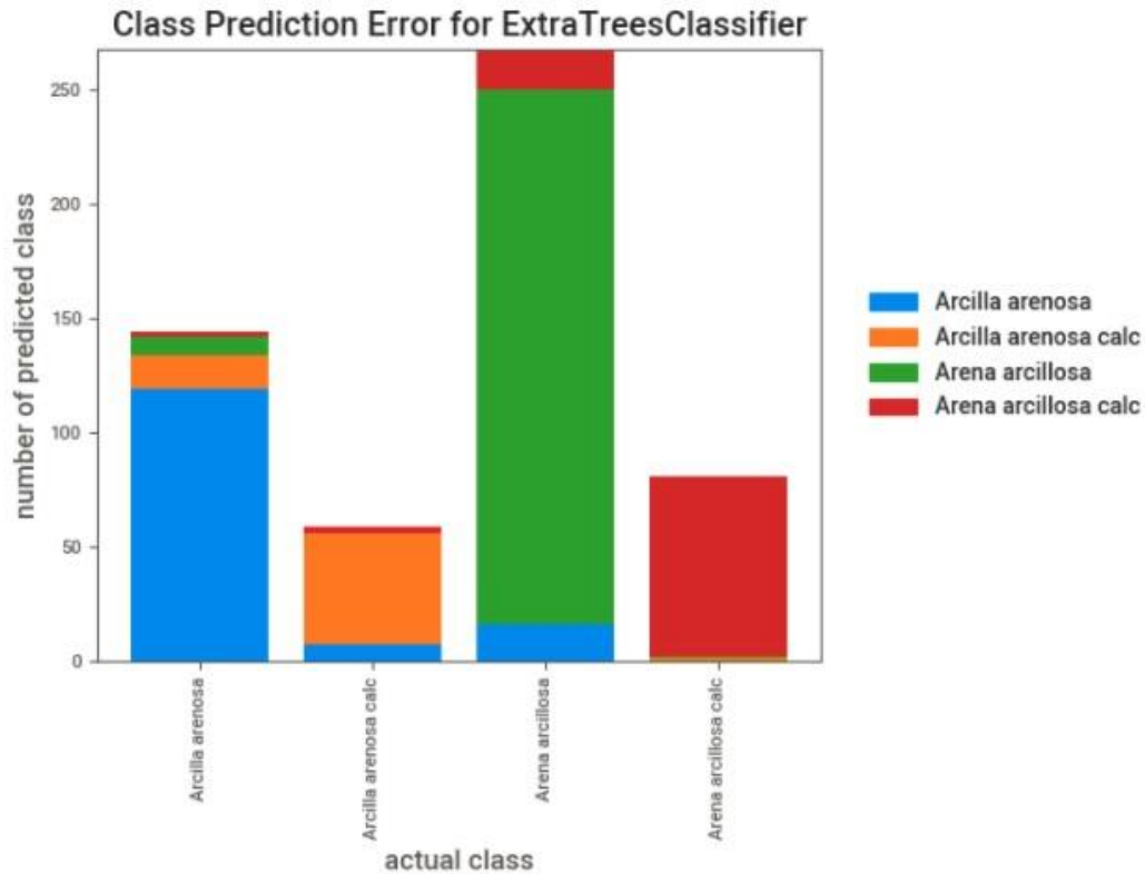
Figura S6. Error de predicción de clase para el Problema 2 . Aunque el modelo parece ser bastante bueno para predecir correctamente las cuatro litologías en función de los registros utilizados, a menudo el modelo etiqueta incorrectamente confundiéndolas con las otras litologías, por ejemplo, cuando es Arcilla arenosa lo puede confundir con Arcilla arenosa calcárea y Arena arcillosa, en menor proporción Arena arcillosa calcárea.
