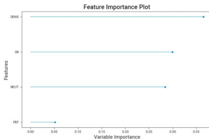
Figura S7. Las categorías utilizadas para el pronóstico del Problema 1 se muestran en orden de importancia. La importancia de cada atributo proporciona una puntuación que indica qué tan útil o valiosa fue cada característica dentro del modelo. En este caso la variable menos importante es PEF.
