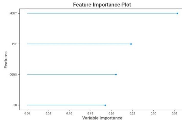
Figura S8. Las categorías utilizadas para el pronóstico del Problema 2 se muestran en orden de importancia. La importancia de cada atributo proporciona una puntuación que indica qué tan útil o valiosa fue cada característica dentro del modelo. En este caso la más importante fue NEUT, pero todas cobran importancia dentro del modelo.
