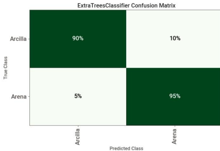
Figura 2. Matriz de Confusión para Problema 1 . Las predicciones muestran un error menor al 10% para ambas clases identificadas.
