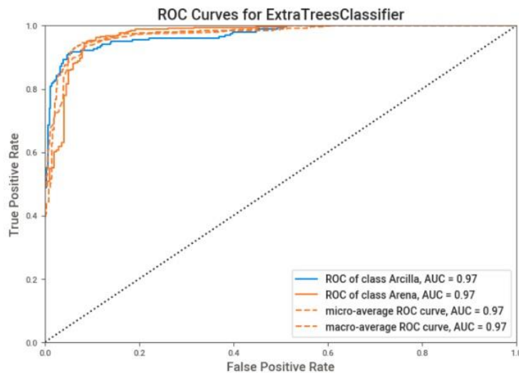
Figura S1. Curva ROC. Para el Problema 1 el área bajo la curva de las dos litologías está dando 0.97.
