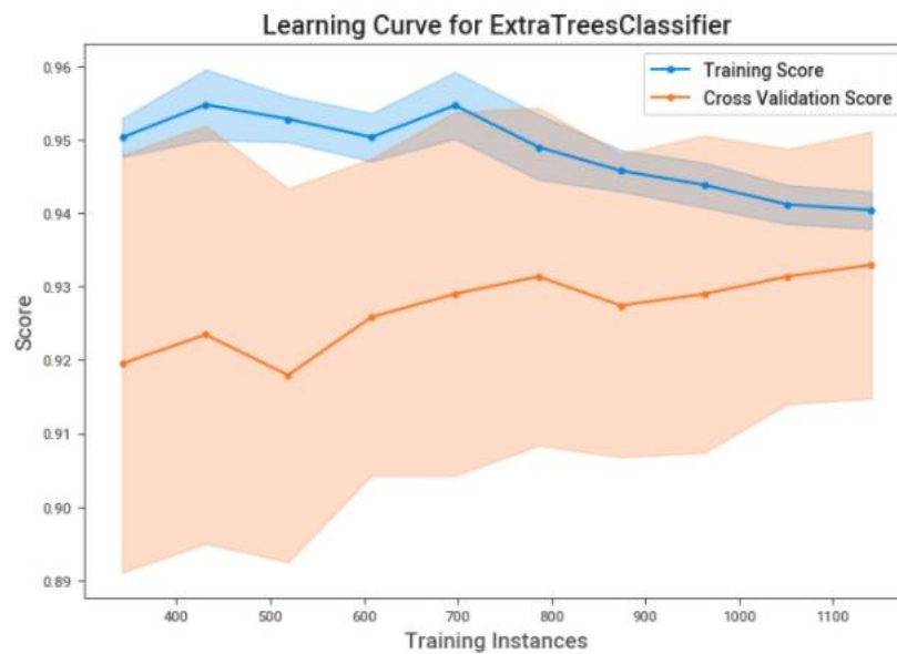
Figura S3. Curva de aprendizaje para el Problema 1 . La línea de valores de entrenamiento se encuentra muy cerca e incluso dentro de la sombra de la línea valores de testeo. El modelo está generalizando de forma correcta.
