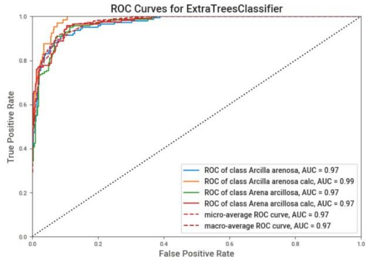
Figura S2. Curva ROC. Para el Problema 2 el área bajo la curva es de 0.97, menos para la categoría de Arcilla Arenosa calcárea que es de 0.99.
