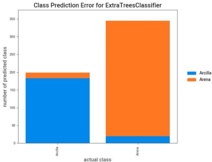
Figura S5. Error de predicción de clase para el Problema 1 . El modelo parece ser bastante bueno para predecir correctamente las litologías de Arena y Arcilla en función de los registros, sin embargo, en pocas ocasiones no etiqueta como debe ser.
