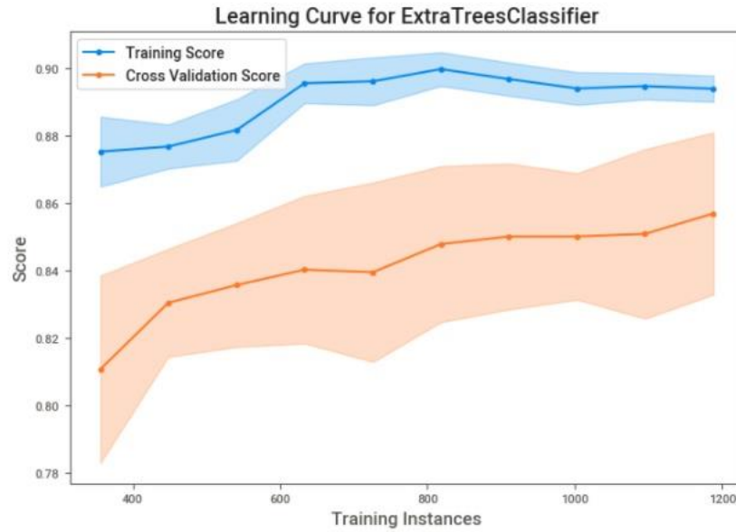
Figura S4. Curva de aprendizaje para el Problema 2 . Las líneas se están acercando, la línea de valores de entrenamiento todavía no alcanza a entrar a la sombra de la línea valores de testeo. El modelo puede mejorar.
